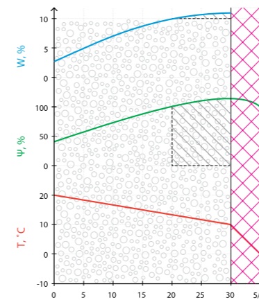
б1 – мокрое утепление по ППС 50 мм
