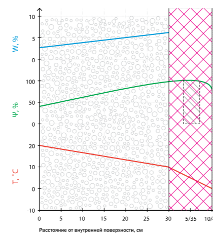
б2 – мокрое утепление по ППС 100 мм
