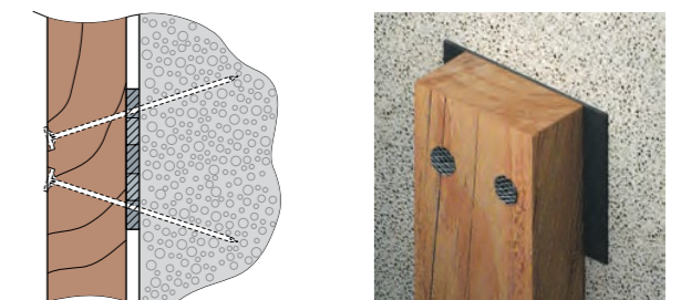
А - деревянная по мокрой кладке
