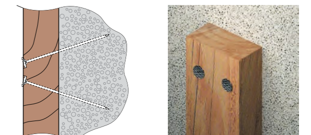
Б - деревянная по сухой кладке
