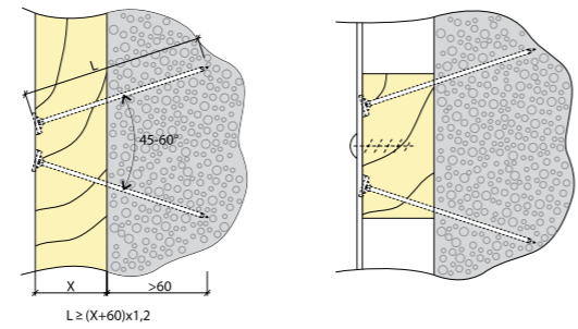
а – деревянный брусок, набитый на кладку непосредственно б – крепление профиля через опорный брусок
