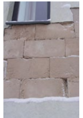
Рис. 16б. Отрыв штукатурки с высоким сопротивлением влагообмену от влажной кладки
