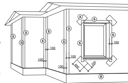
Рис. 15. Схема армирования штукатурки
