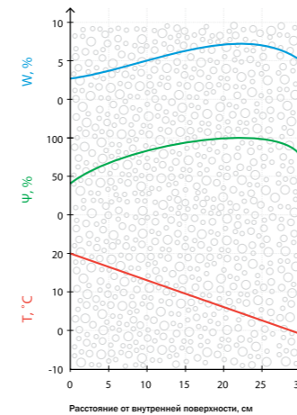
а – однослойная кладка
