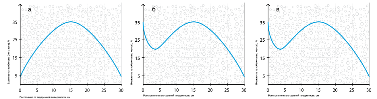
Рис. 19. Распределение влаги по толщине стены. Стена здания с незакрытым контуром через месяц после кладочных работ
