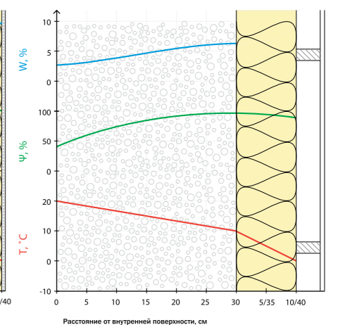
г2 – минвата и облицовка на отnose
