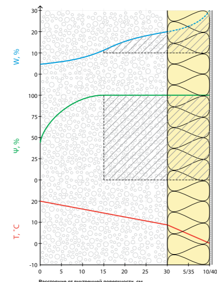
в2 – мокрое утепление по минвате 100 мм
