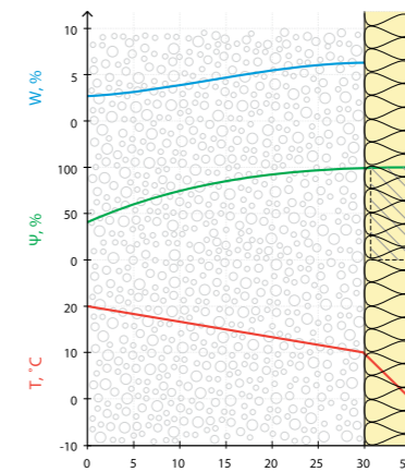
в1 – мокрое утепление по минвате 50 мм
