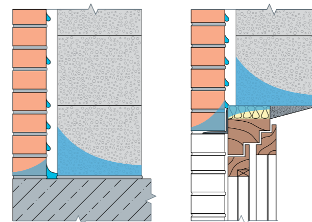
А – в зоне опирания облицовки на цоколь
