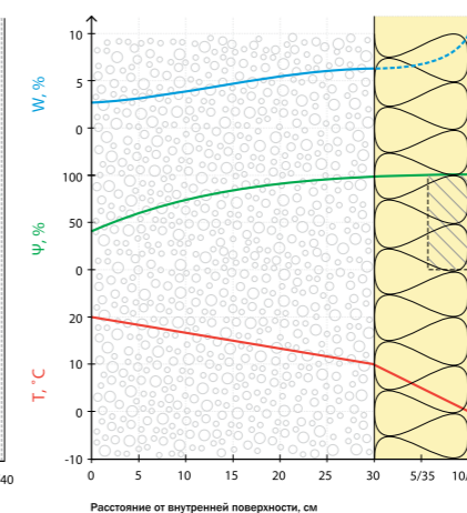
в2 – мокрое утепление по минвате 100 мм
