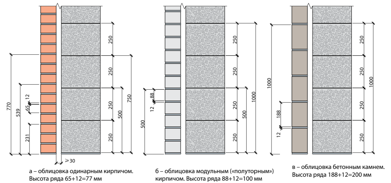
Рис. 13. Двухслойные кладки с облицовками
