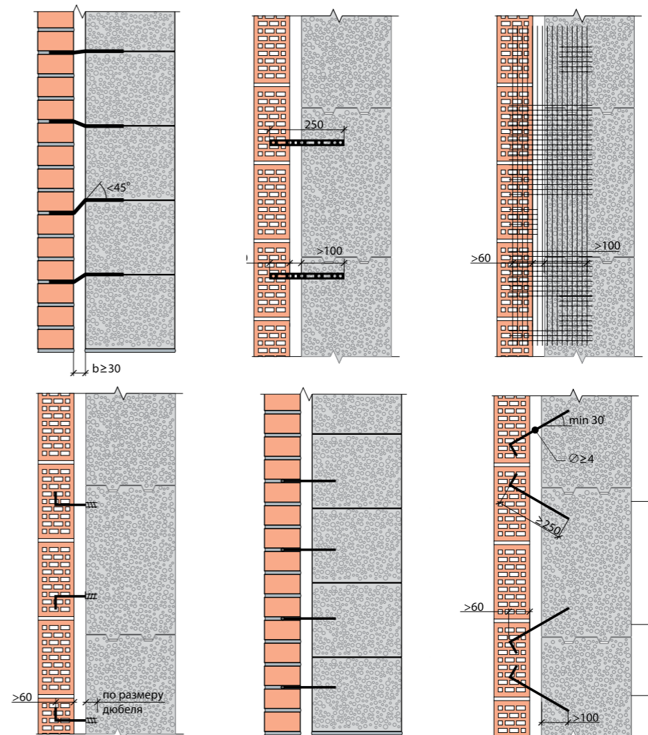
Рис. 14. Связь облицовочного и основного слоев кладки
