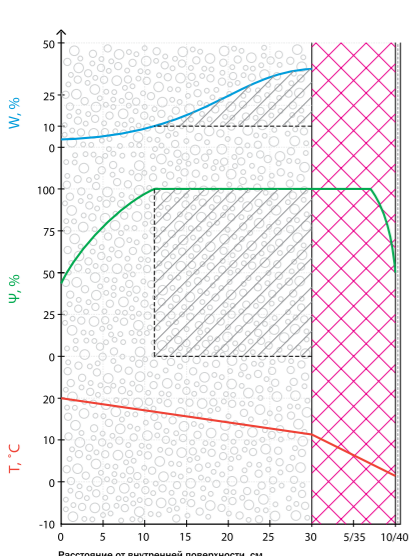
б2 – мокрое утепление по ППС 100 мм
