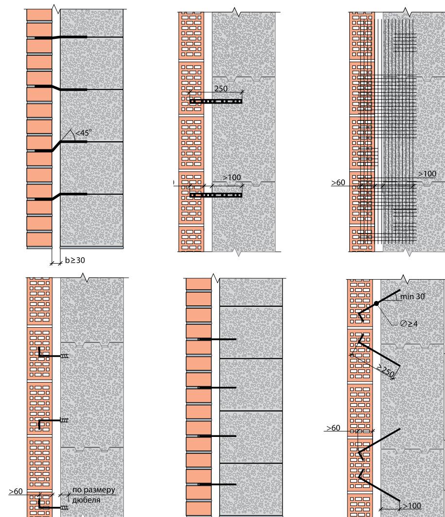
Рис. 14. Связь облицовочного и основного слоев кладки
