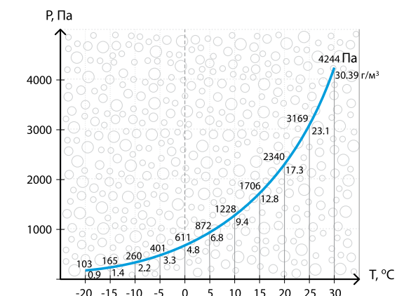
Рис. 23. Давление насыщения водяного пара и максимальное содержание водяного пара в воздухе в зависимости от температуры
