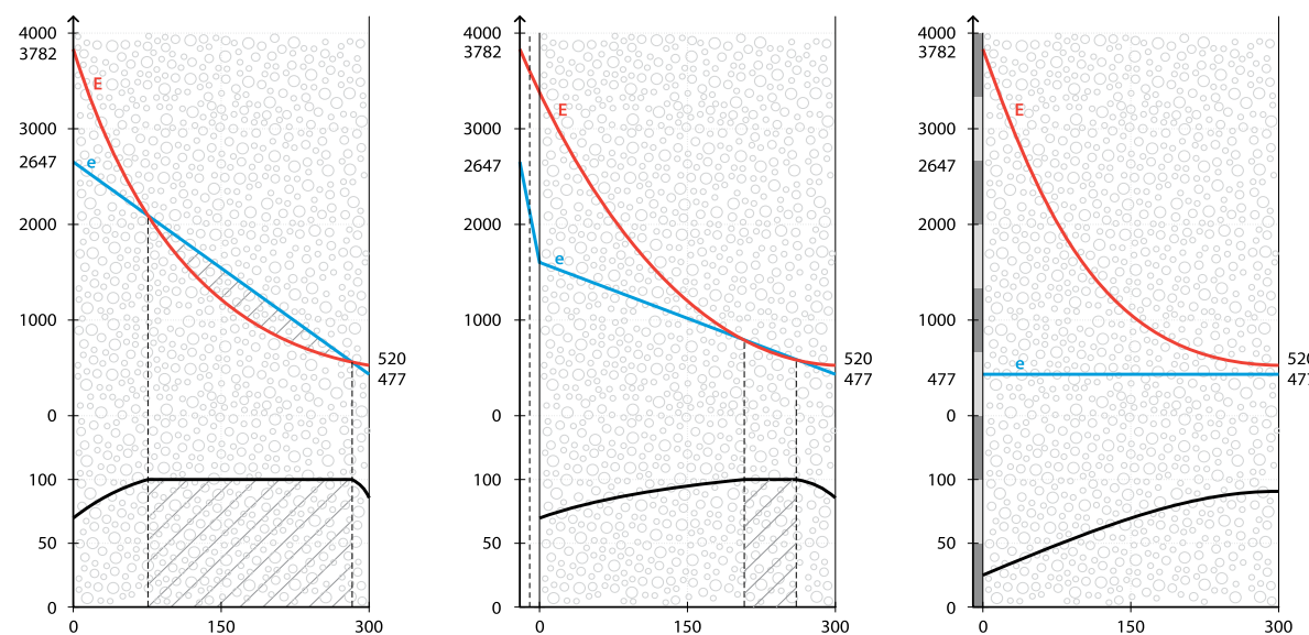
Рис. 26. Влияние внутренней пароизоляции на распределение влажности воздуха в порах по толщине стены.
