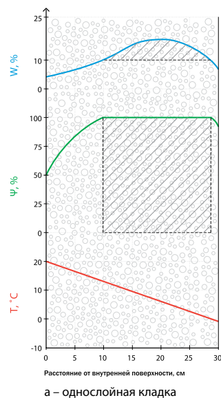
Рис. 21. Распределение влаги, температуры и давления водяного пара по толщине стены в отопительный период. Начальная влажность газобетона – 100 кг/м 3 (25 % для D400, 20 % для D500, 15 % для D600). Заштрихованная область – зона, в которой влажность газобетона выше сорбционной, зона возможной конденсации.
