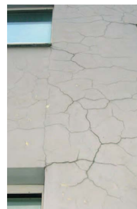
Рис. 16а. Трещины на штукатурке, затворенной избытком воды
