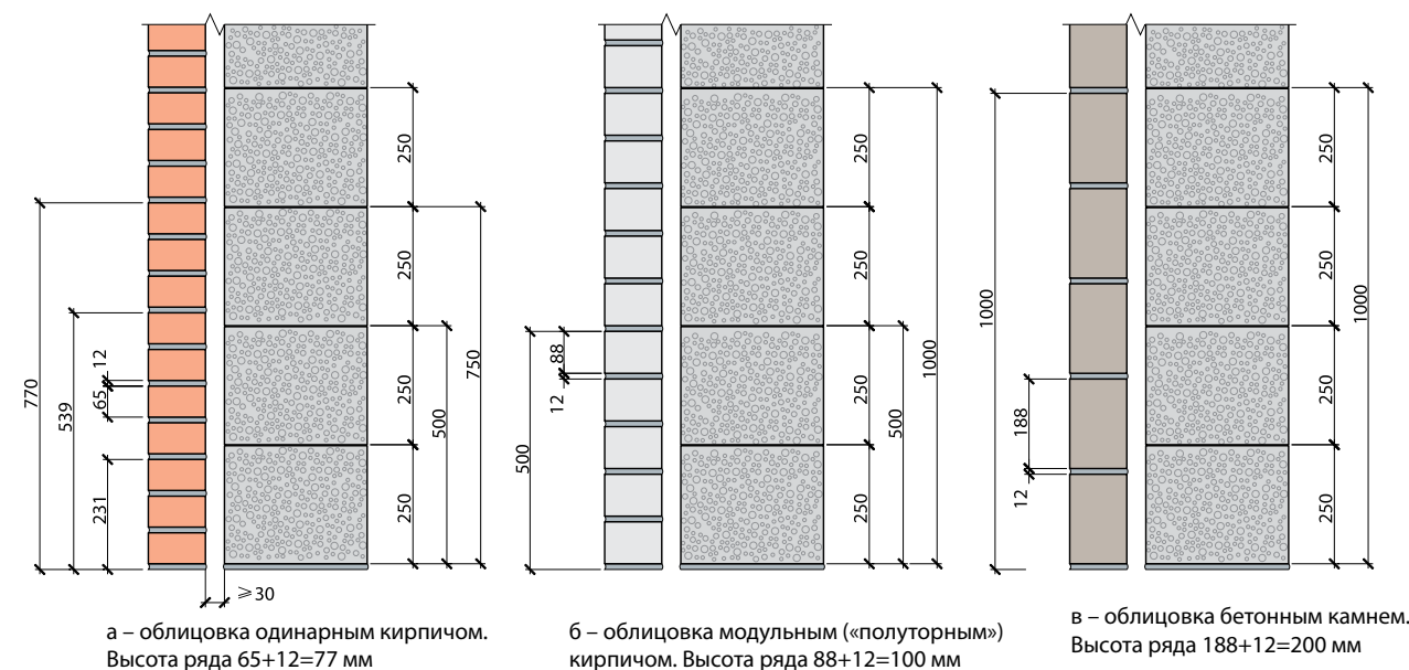
Рис. 13. Двухслойные кладки с облицовками
