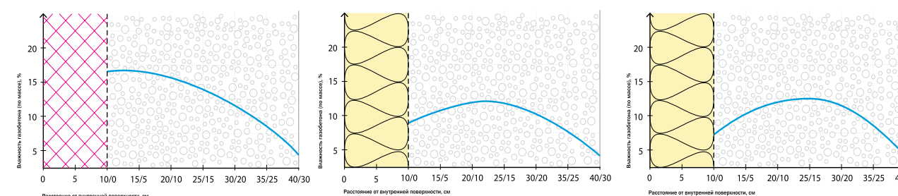
Рис. 20. Распределение влаги по толщине утепленной стены. Стена здания с незакрытым контуром через четыре месяца после кладочных работ
