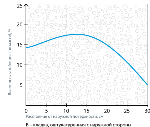
Рис. 5. Влияние дождей и штукатурки на влажность газобетона (стена из D400 через полгода после кладки)
