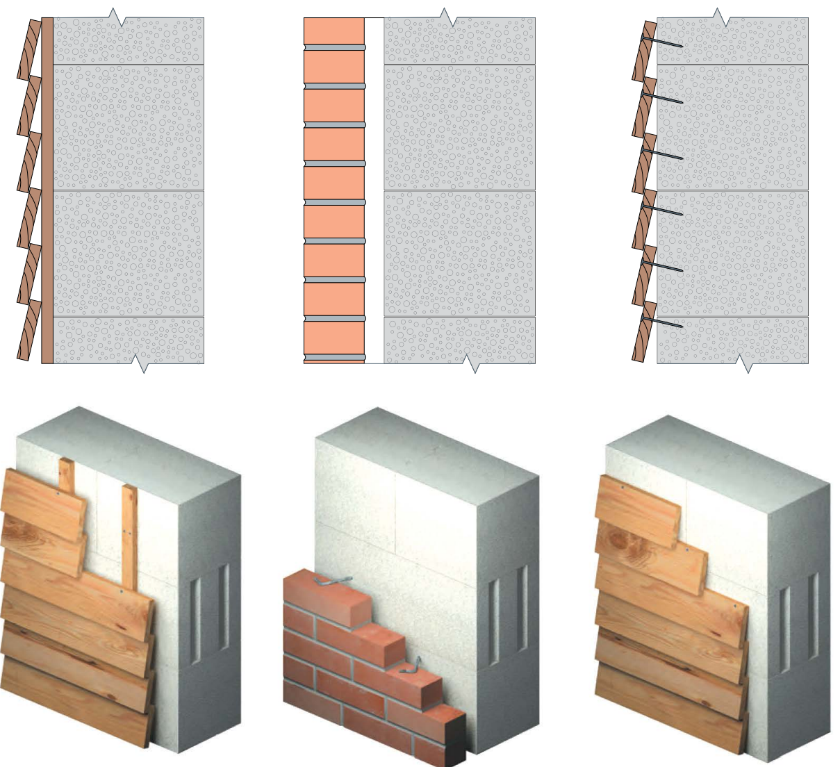
Рис. 7а. Облицовка по направляющим
