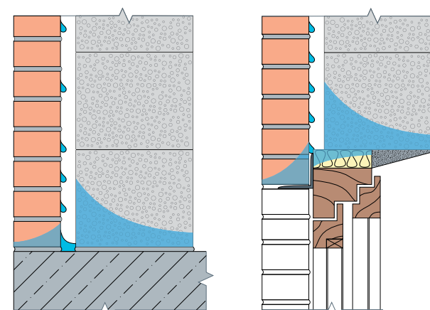
Рис. 8. Конденсат на внутренней поверхности облицовки. Зона потенциального увлажнения
