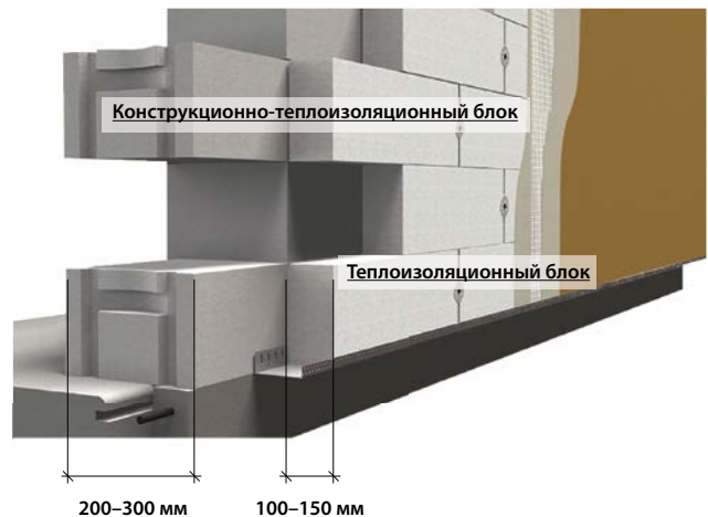
Рис. 4. Энергоэффективные двухслойные стены из газобетона с внешним утеплением ЛСР ТЕРМО
