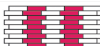
Ложковая кладка
