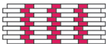
Готическая кладка
