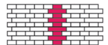
Крестовая кладка
