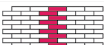
Ложковая кладка
