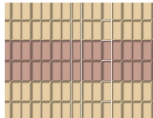
«Паркетная» укладка на тычок
