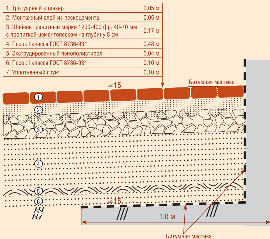
Рисунок №4. Гидроизоляция подземных частей зданий, к которым примыкает мощение
