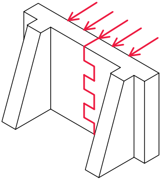
Рис. 3.3. Растяжение кладки при изгибе по перевязанному сечению
