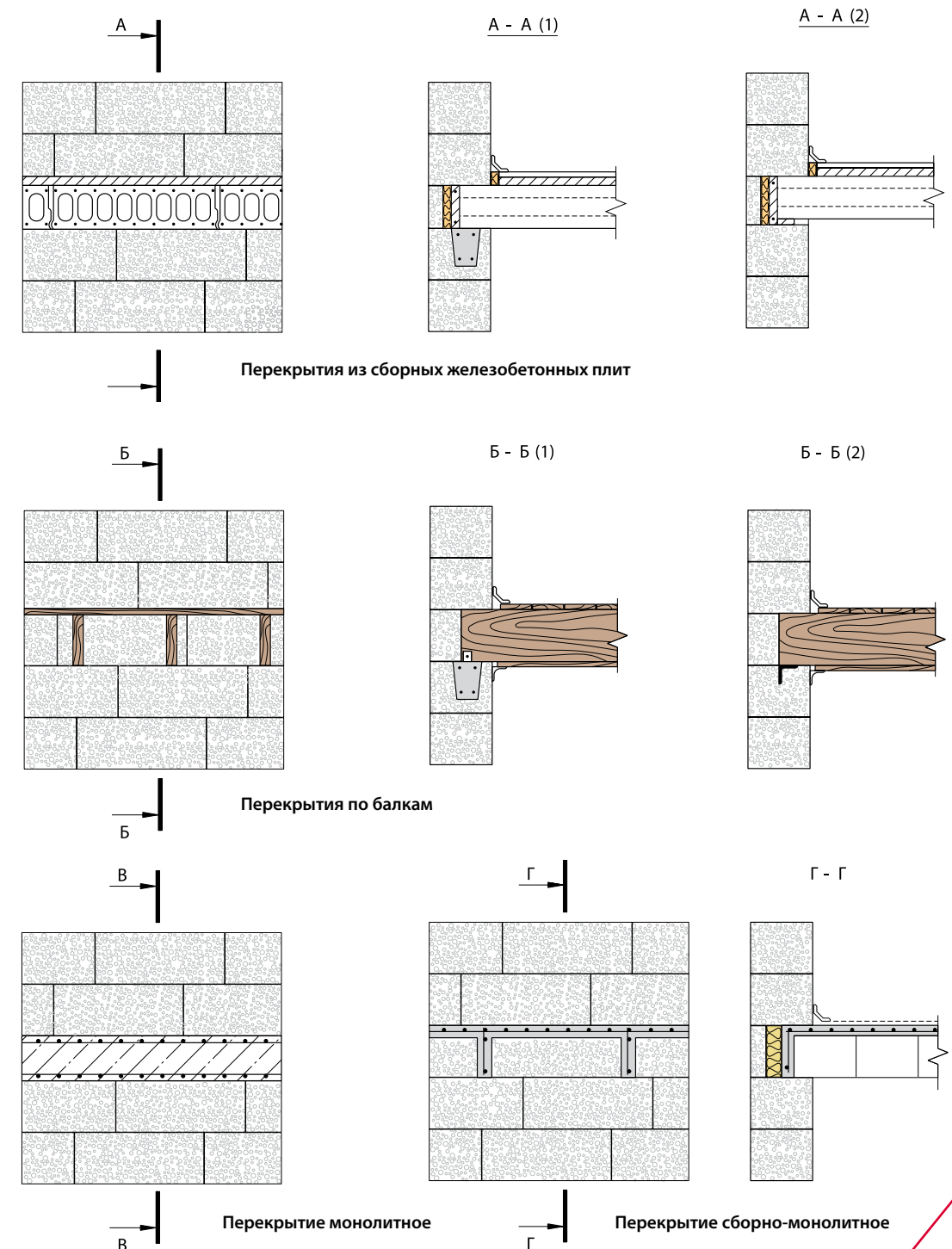
Рис. 4.11. Варианты перекрытий по стенам из блоков
