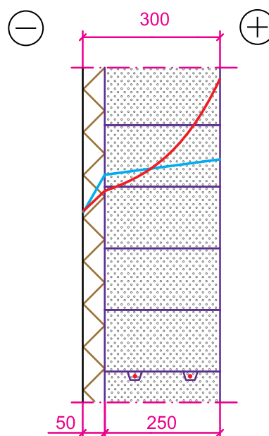
Наружное утепление пенополистиролом: конденсация возможна на границе [несущая стена/утеплитель]
