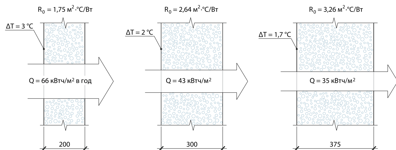
Рис. 1. Увеличение толщины стен сверх 200 мм мало влияет на комфорт, но уменьшает теплотери при постоянном отоплении
