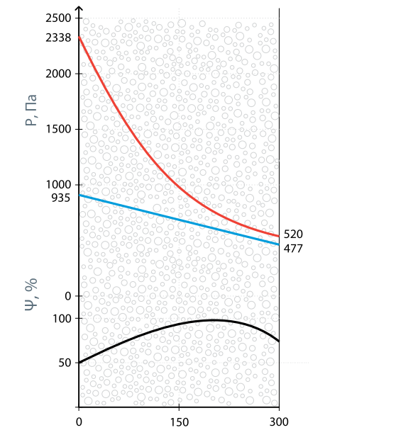
Давление реального и насыщенного водяного пара в толще стены красная – кривая распределения насыщенного пара; голубая – кривая распределения реального пара по толщине стены; черная – кривая распределения влажности воздуха в порах.
