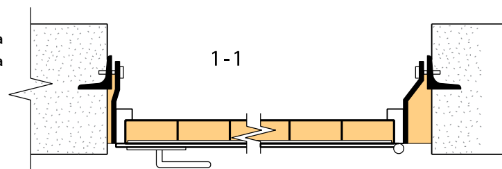
Рис. 4.10. Крепление дверного блока с большой массой полотна
