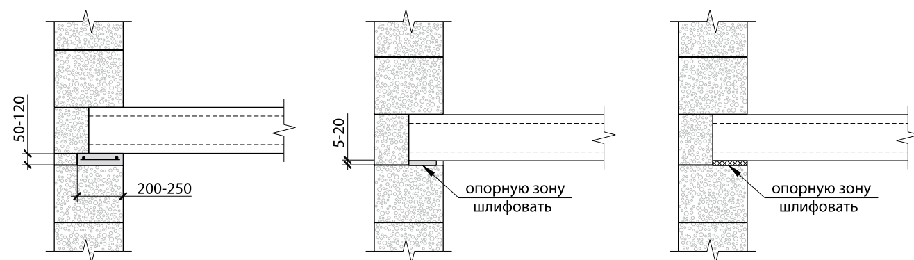
Рис. 4.13. Варианты перекрытий по стенам из блоков ЛСР
