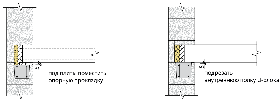
Рис. 4.12. Варианты перекрытий по стенам из блоков ЛСР
