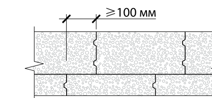
Рис. 4.4. Перевязка кладки
