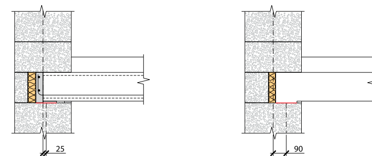
А – увеличение глубины опирания и включение в работу связочного пояса
